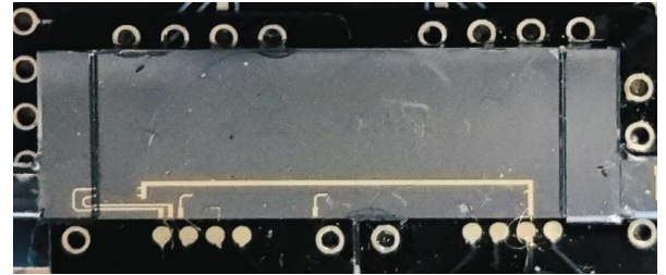
图 4 非对称马赫-曾德尔干涉仪实物图
