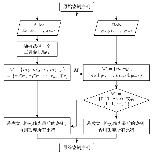
图 1 优势提纯方法的流程图
