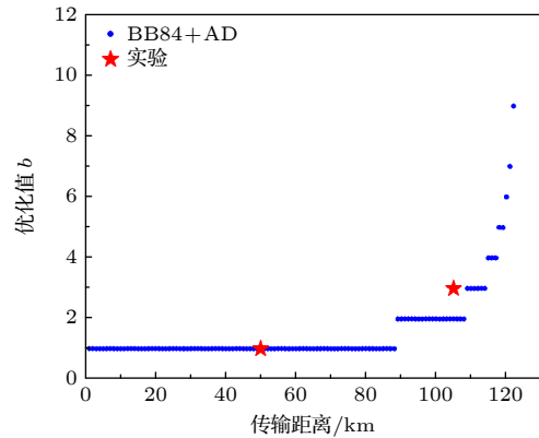
图 6 基于 AD 技术的 BB84 协议的理论最优值 b
