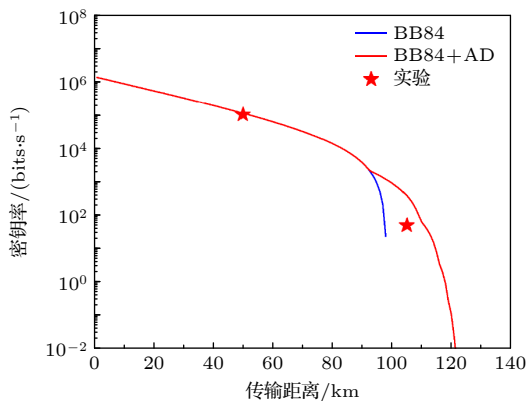
图 5 基于 AD 技术的 BB84 协议的理论密钥率对比图
