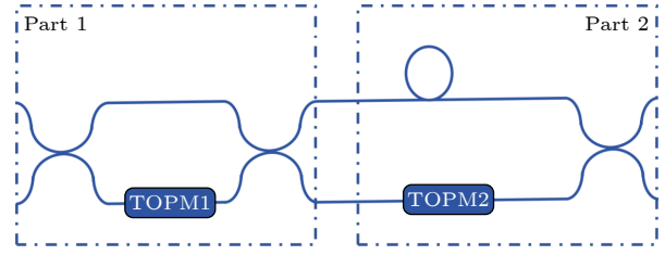
图 3 非对称马赫-曾德尔干涉仪原理图
