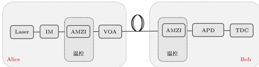
图 2 BB84 QKD 系统实验装置结构示意图, 其中 Laser 为激光器模块, IM 为强度调制器, AMZI 为非对称马赫-曾德尔干涉仪, APD 为探测器模块, TDC 为时间数字转换器
