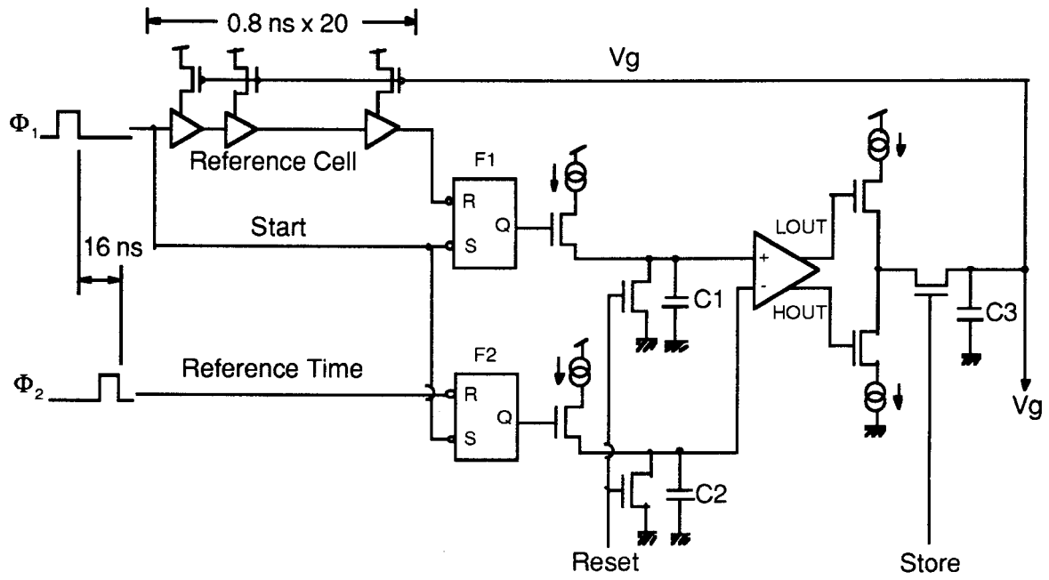
Fig. 5 TMC Feedback Circuit.
