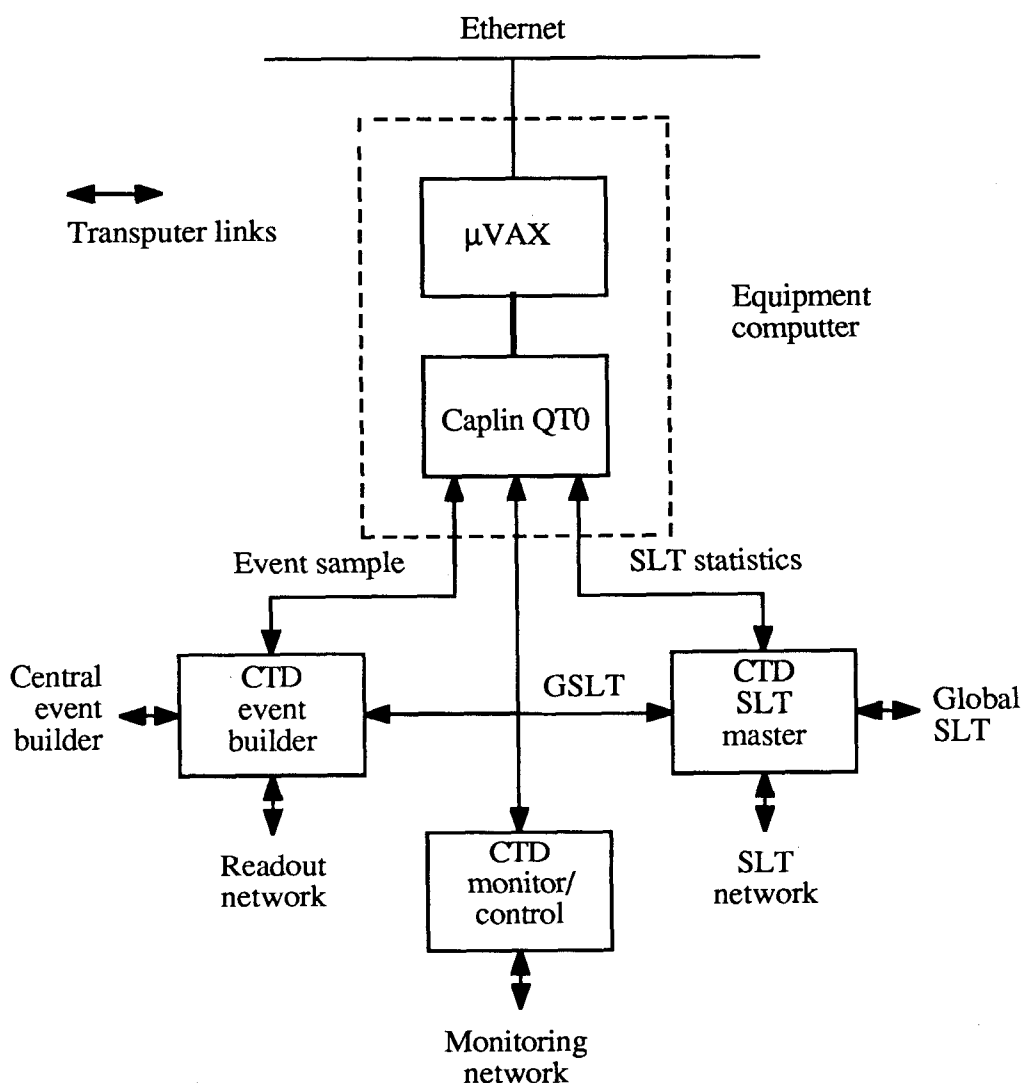
Fig 3. Detector readout
