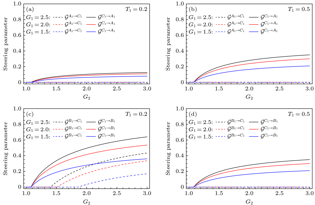
图 2 在不同透射率 T_1 和增益 G_1 下, 两模间的量子导引参数随 G_2 的变化 (a) T_1 = 0.2 时, 模 \hat{A}_1 和 \hat{C}_1 之间的导引; (b) T_1 = 0.5 时, 模 \hat{A}_1 和 \hat{C}_1 之间的导引; (c) T_1 = 0.2 时, 模 \hat{B}_1 和 \hat{C}_1 之间的导引; (d) T_1 = 0.5 时, 模 \hat{B}_1 和 \hat{C}_1 之间的导引
