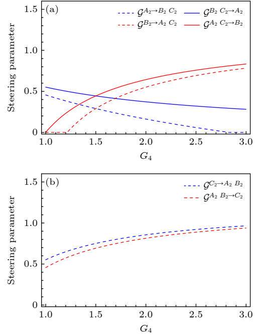
图 7 一个模式与另外两个模式之间的量子导引参数随增益 G_4 的变化 ( G_1 = G_2 = 2 ): (a) 模式 \hat{A}_2 和 \hat{B}_2 分别作为导引方和被导引方; (b) 模式 \hat{C}_2 作为导引方和被导引方
