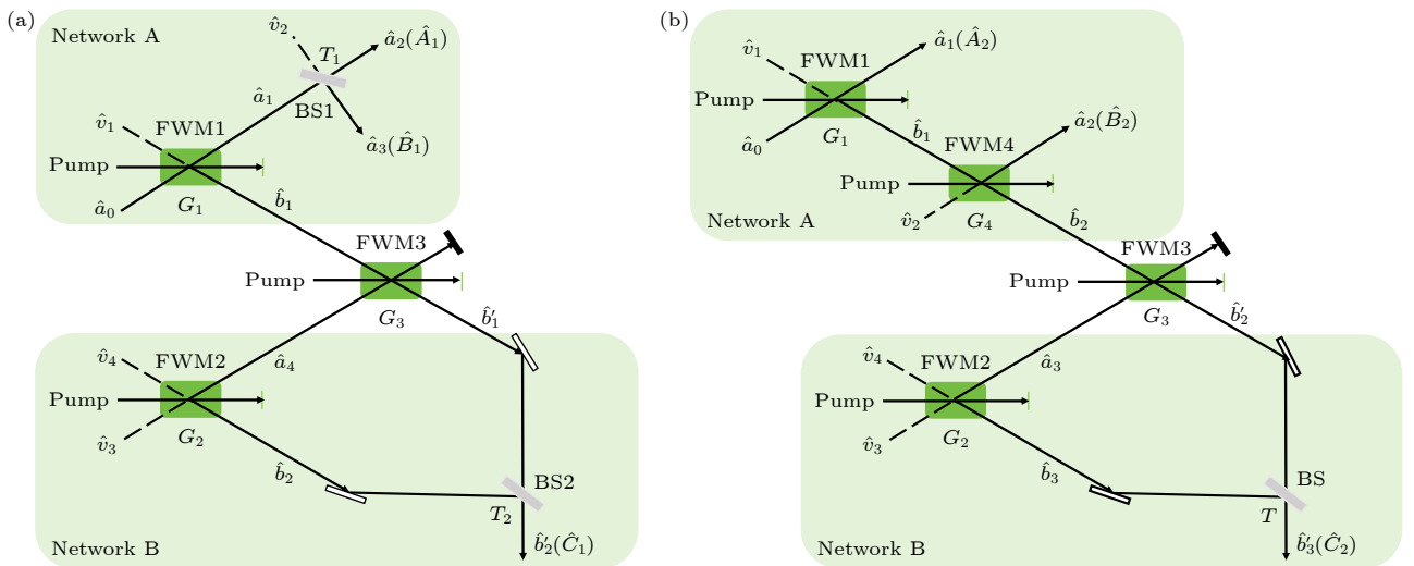
图1 三组份全光量子导引交换方案示意图 (a) 利用线性分束器方案; (b) 利用非线性分束器方案
