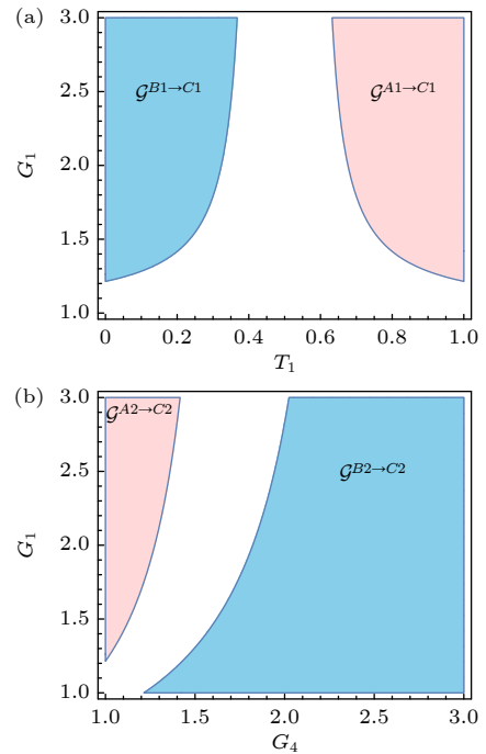
图 8 单配性关系的操控 ( G_2 = 2 ) (a) 线性分束器方案; (b) 非线性分束器方案
