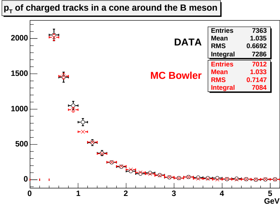
Figure 7: Comparaison entre données et simulation, contenant tous mécanismes de production du quark b . La distribution de l'impulsion transverse au faisceau des traces dans un cône défini autour du B
