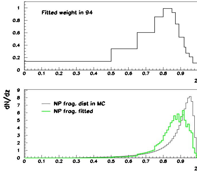
Figure 2: Distributions, en fonction de la variable z , obtenues pour les événements sélectionnés en 1994. En haut: Distribution fittée des poids. En bas: Comparaison entre la distribution de Peterson utilisée dans le générateur et la distribution fittée sur les données.
