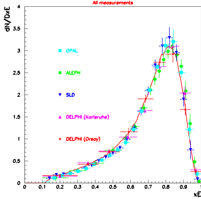
Figure 3: Comparaison entre les distributions de la variable x_E mesurées par ALEPH, DELPHI, OPAL et SLD.
