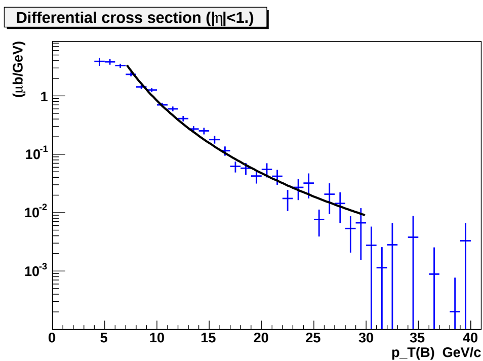
Figure 8: La section efficace différentielle de production du quark b avec pseudo-rapidité inférieure à 1.
