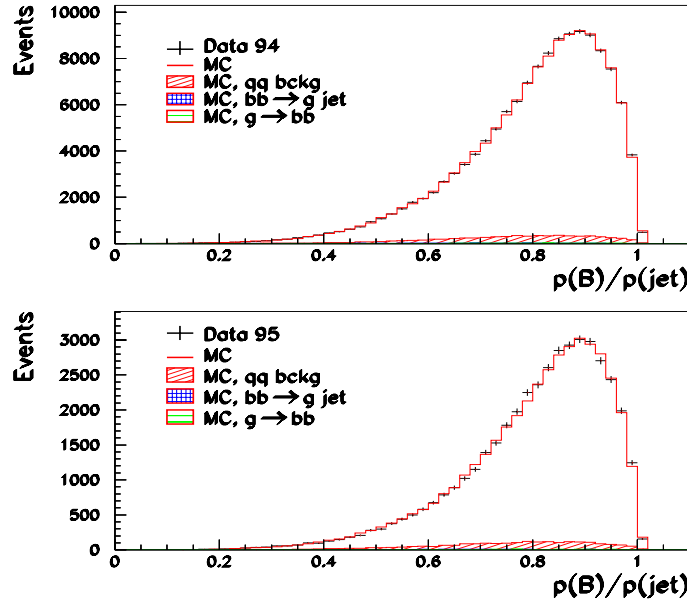
Figure 1: Distributions fittées, en fonction de x_p^{rec} = p_B^{rec} / p_{jet} , pour les événements sélectionnés. En haut: échantillon 1994. En bas: échantillon 1995.
