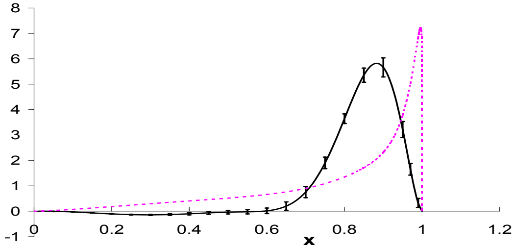
Figure 4: La distribution de la composante QCD non-perturbative de la fonction de fragmentation du quark b , obtenue à partir des mesures effectuées dans DELPHI, à l'occasion de cette thèse, et en utilisant le générateur JETSET pour évaluer la composante QCD perturbative.
