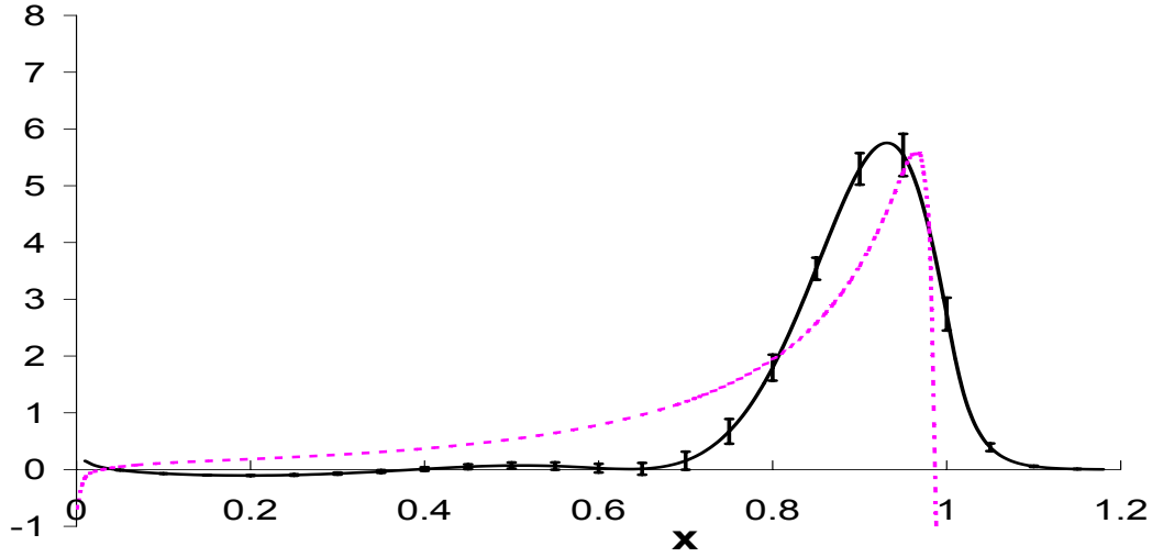
Figure 5: La distribution de la composante QCD non-perturbative de la fonction de fragmentation du quark b , obtenue à partir des mesures effectuées dans DELPHI, à l'occasion de cette thèse, et en utilisant un calcul analytique basé sur QCD à l'ordre NLL pour évaluer la composante QCD perturbative.
