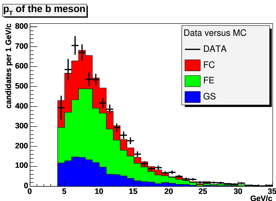
Figure 6: Comparaison entre données et simulation, contenant tous mécanismes de production du quark b . La distribution de l'impulsion transverse au faisceau du méson-B. Les contributions des différents mécanismes de production du B sont montrés séparément les uns des autres.
