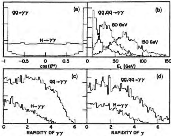
Fig. XII.2: Distributions of (a) \cos\theta^* , (b) E_T^\gamma , (c) \eta_\gamma , and (d) \eta_\gamma .
