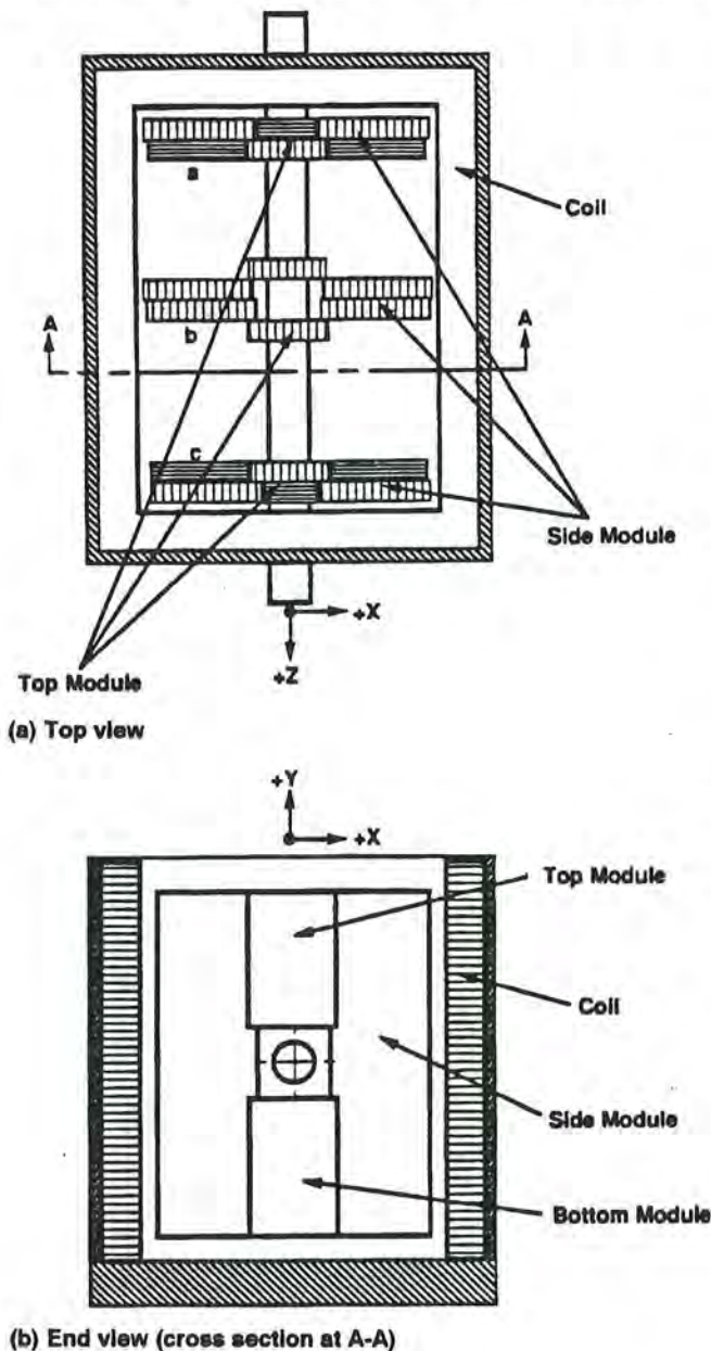
Fig. IV.30. Forward muon detector.
