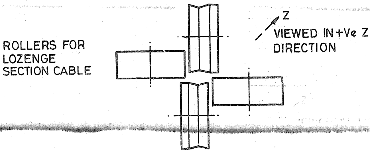
FIG. 8. TURKSHEAD ROLLER DIE
