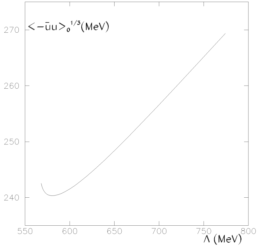
Figure 4.2 - Valeur du condensat de quarks dans le vide (1 saveur) ( -\langle \bar{u}u \rangle_0 ) 1/3 en fonction de \Lambda .
