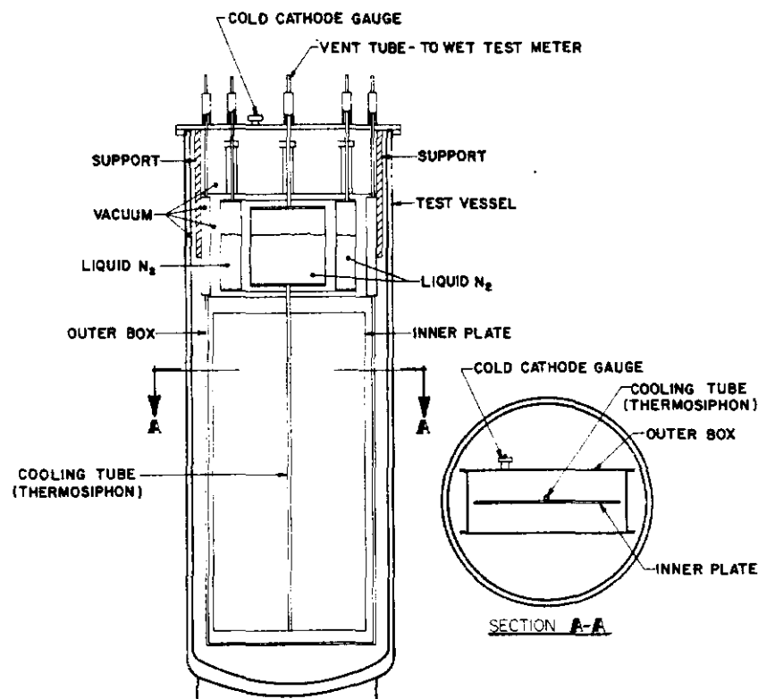
Fig. 1. Test apparatus.
