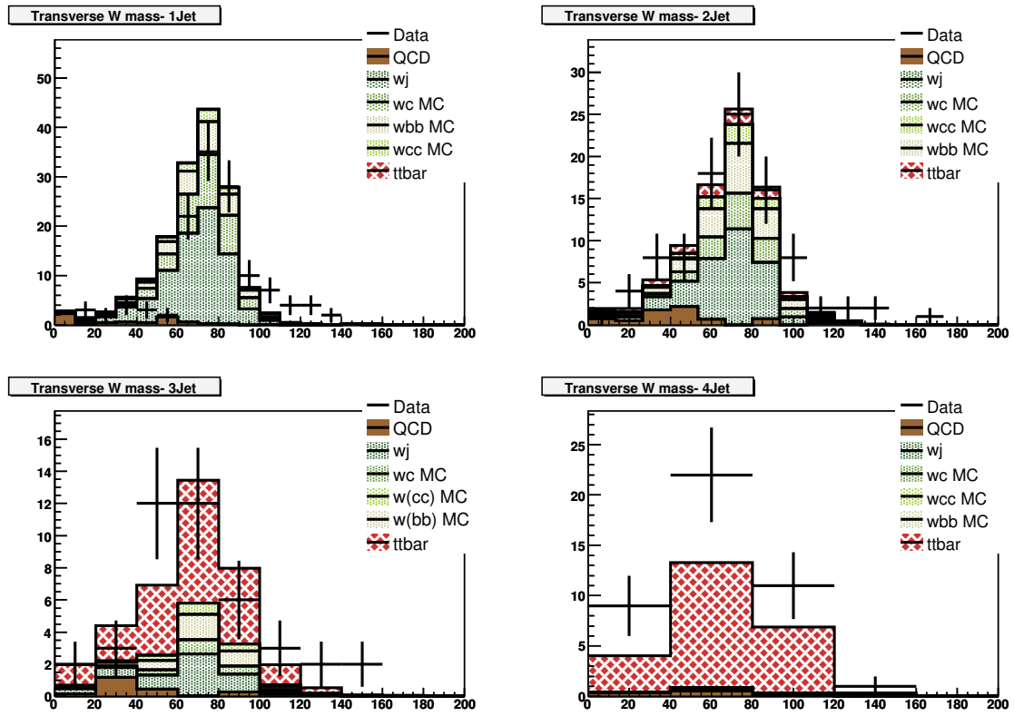
Fig. A.12. e+jets : W boson transverse mass.
