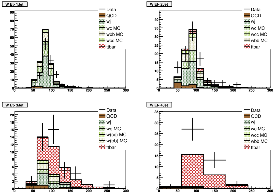
Fig. A.13. e^+ \text{jets} : W boson E_T .
