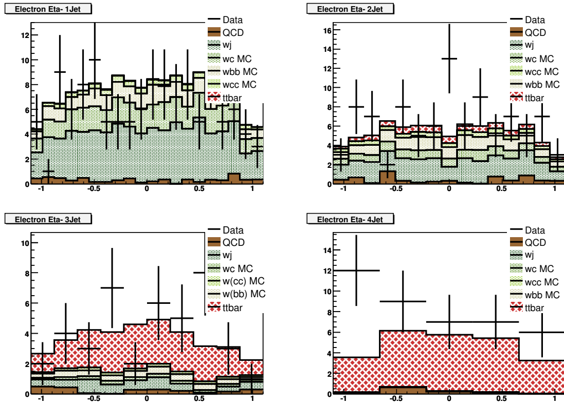
Fig. A.6. e +jets: electron |\eta| .
