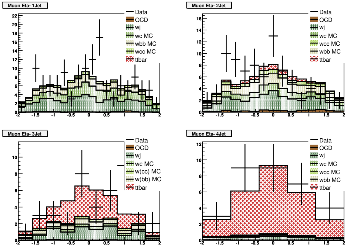
Fig. A.20. \mu +jets: muon |\eta| .
