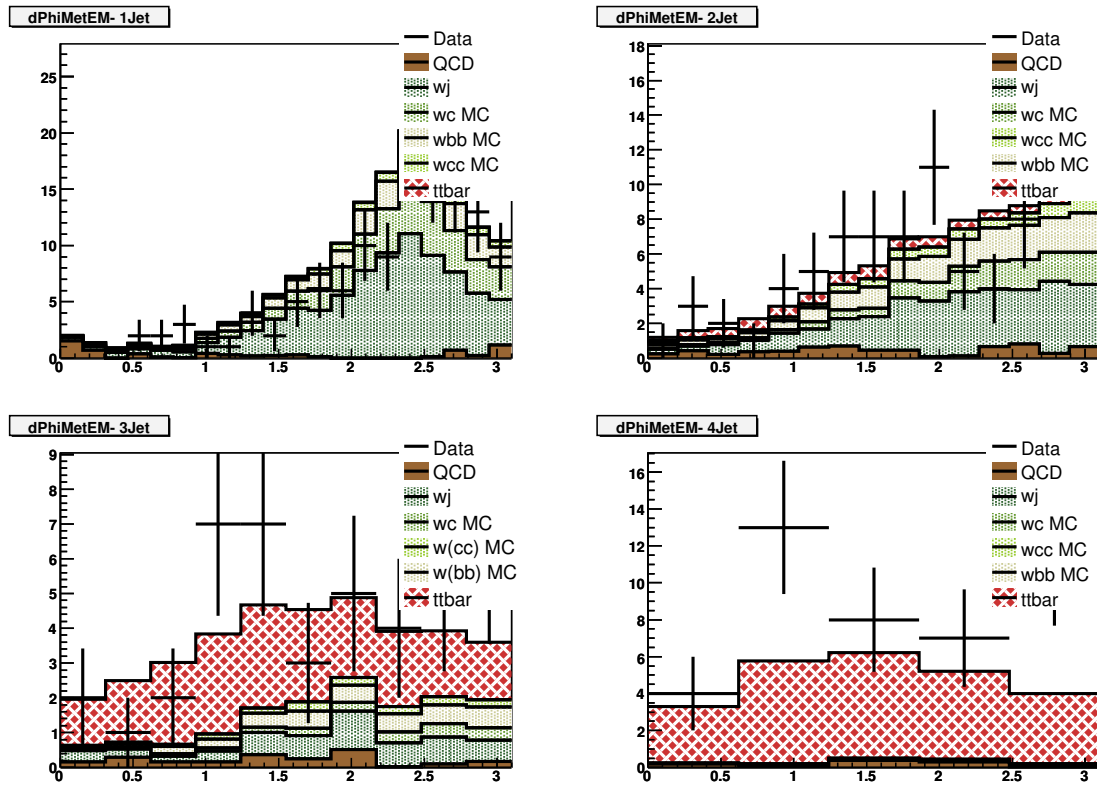
Fig. A.5. e+\text{jets} : \Delta\phi(\text{electron}, \text{missing } E_T) .
