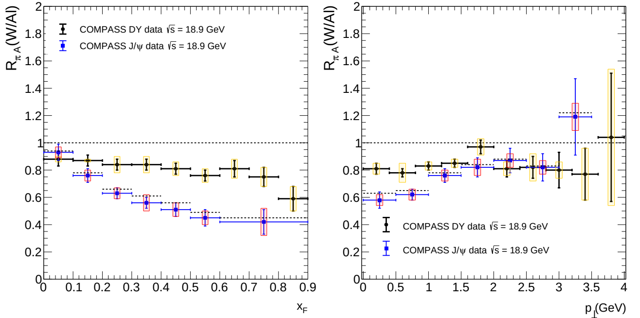
Figure 6: Rapport des sections efficaces dans les collisions \pi^- W et \pi^- Al pour les processus Drell-Yan (en noir) et J/\psi (en bleu) incluant les erreurs statistiques (ligne) et systématiques (rectangle).
