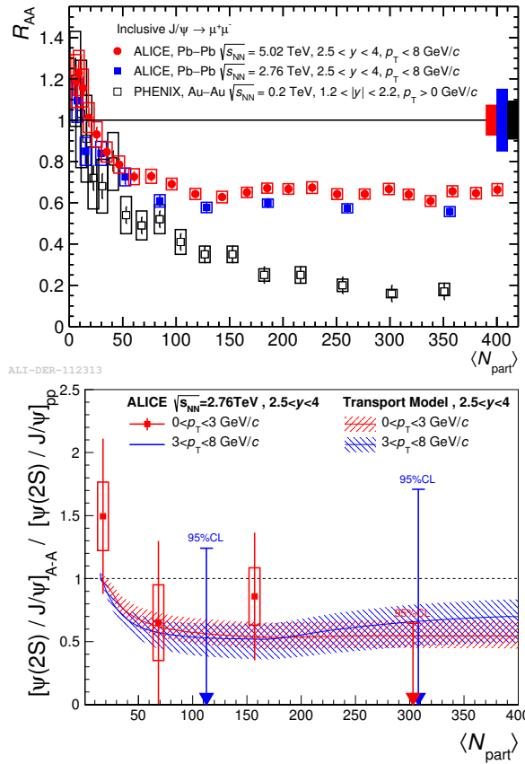
FIGURE 2: Haut : Facteur de modification nucléaire inclusif du J/\psi en fonction du N_{\text{part}} mesuré dans des collisions Pb – Pb à \sqrt{s_{NN}} = 2.76 TeV et \sqrt{s_{NN}} = 5.02 TeV comparé aux mesures de PHENIX dans des collisions Au – Au à \sqrt{s_{NN}} = 0.2 TeV [26, 27]. Bas : Double rapport en fonction de N_{\text{part}} mesuré dans des collisions Pb – Pb à \sqrt{s_{NN}} = 2.76 TeV [26].
