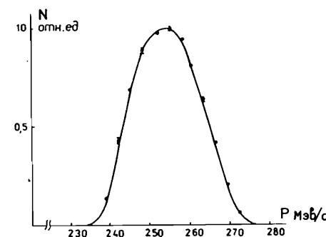
Рис.3. Импульсный спектр α-частиц.
