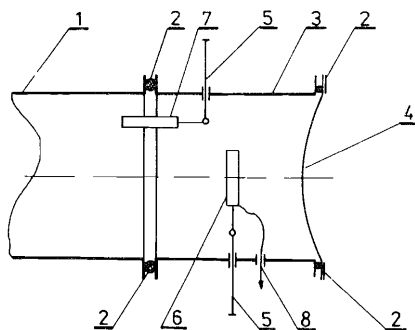
Рис.1. Схема камеры с ППД: 1 - труба вакуумпровода, 2 - уплотнения, 3 - корпус камеры, 4 - майларовая пленка, 5 - шток, 6 - ППД, 7 - α-источник, 8 - вывод сигнала с ППД.
