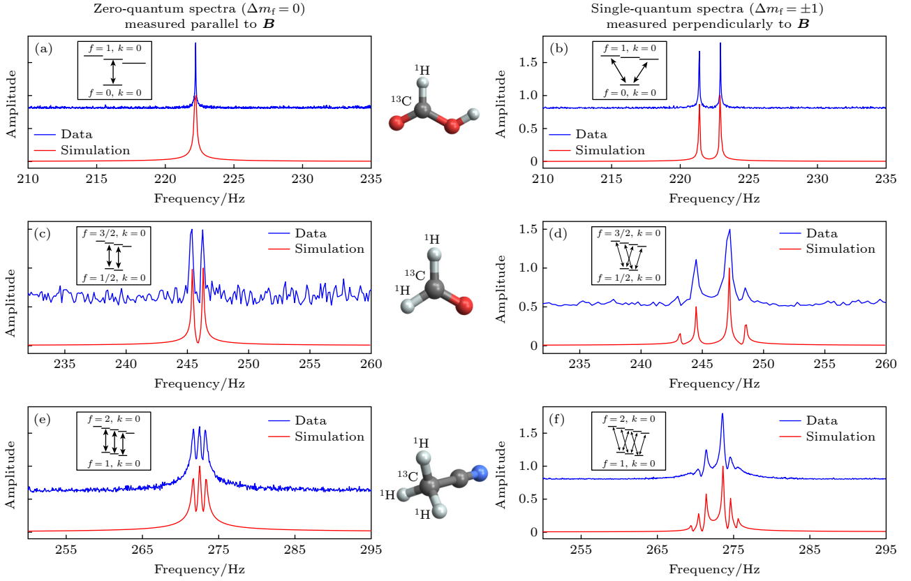
图 2 在不同方向磁场下测量的 ^{13}\text{CH}_n 分子谱学 (a), (b) ^{13}\text{C} -甲酸; (c), (d) ^{13}\text{C} -甲醛; (e), (f) ^{13}\text{C} -乙腈. 分裂模式与插图中显示的跃迁高度匹配
