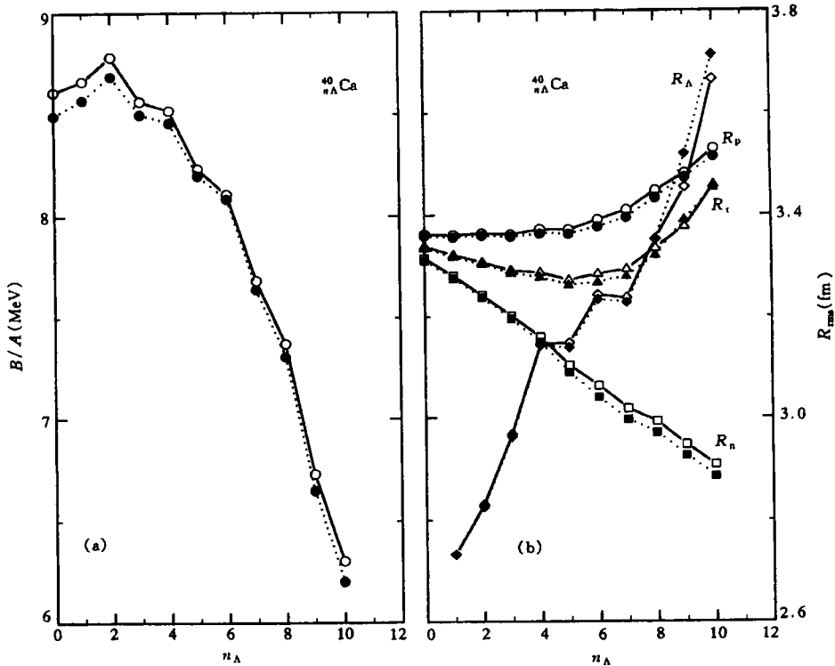
图 3 Ca 的另一种多 \Lambda 超核的基态性质
