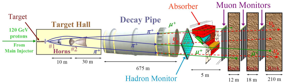
Fig. 1. The NuMI beam-line [1].
