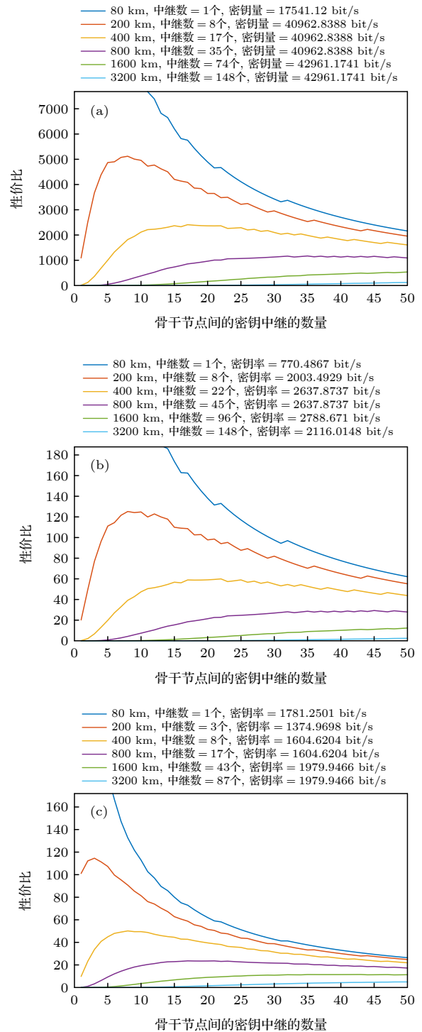
图 6 (a) 采用 BB84 协议时不同距离下中继数量与性价比关系图; (b) 采用 MDI 协议时不同距离下中继数量与性价比关系图; (c) 采用 TF 协议时不同距离下中继数量与性价比关系图
