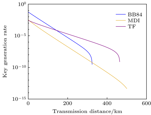
图 5 3种协议密钥产生速率随距离变化曲线图
