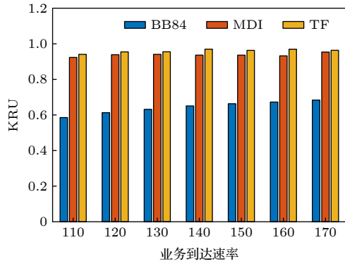
图 9 密钥利用率随业务到达速率变化曲线
