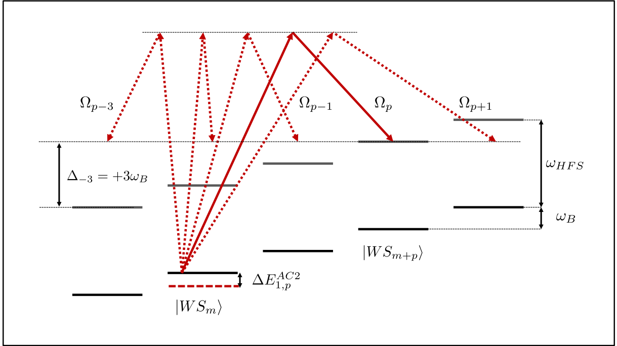
FIGURE III.10 – Déplacement lumineux différentiel à deux photons pour une échelle de Wannier-Stark . Lors d'une transition \Delta m = p , la paire de faisceaux Raman induit plusieurs couplages non-résonnants avec l'ensemble des états de Wannier-Stark |WS_i\rangle désaccordés de \Delta = (i - p) \times \omega_B . La transition résonnante est alors décalée d'une quantité \Delta E_{1,p}^{AC2} . Par soucis de simplicité, seul le déplacement de l'état |WS_m, F = 1\rangle a été représenté, l'état |WS_{m+p}, F = 2\rangle étant déplacé d'une même quantité dans le sens opposé.
