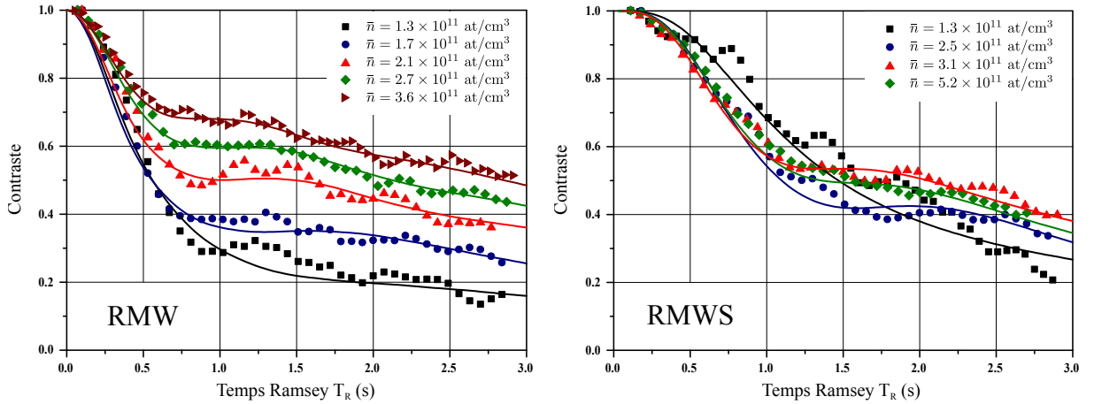
FIGURE IV.10 – a) Contraste des interféromètre Ramsey micro-onde (RMW) et Ramsey-Raman avec \Delta m = 0 (RR0). b) Contraste des inteféromètres symétriques RMWS et RRS0.
