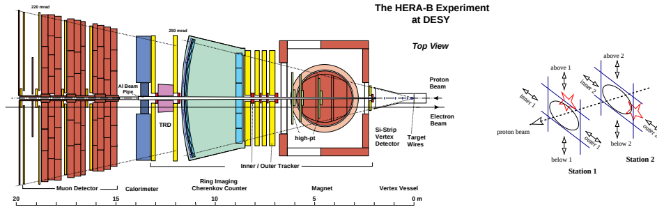
Fig. 1. HERA-B detector.
