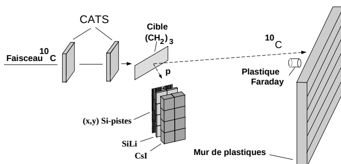
FIG. 2.2 – Montage expérimental
