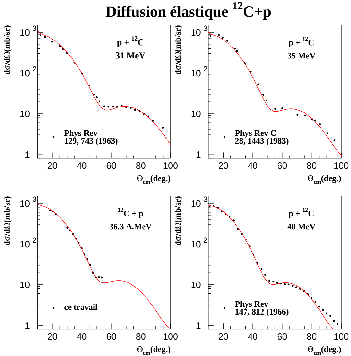
FIG. 3.27 – Comparaison entre des résultats expérimentaux et des calculs utilisant le potentiel d'interaction microscopique complexe nucléon-noyau JLM
