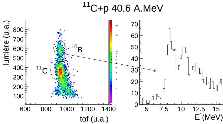
FIG. 3.17 – Matrice de corrélation ( \theta_{lab}^p; E_{lab}^p ) et spectre en énergie d'excitation du ^{11}\text{C} pour la réaction ^{11}\text{C} + p à 40.6 A.MeV avec la sélection du ^{10}\text{B} dans les platiques scintillants.
