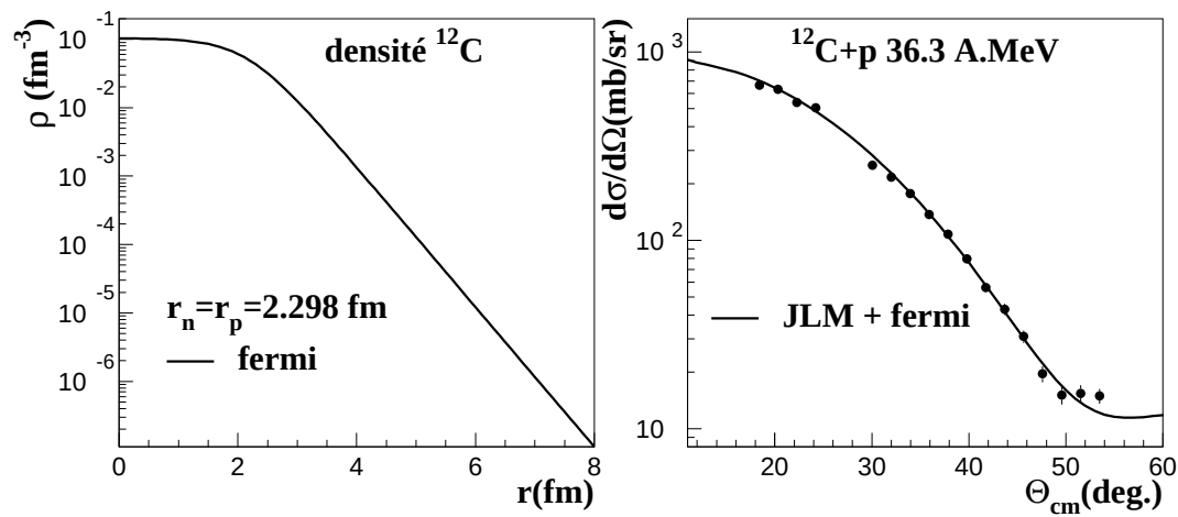
FIG. 4.3 – Densité de Fermi de l'état fondamental [92] et comparaison entre les données mesurées lors de cette expérience et le calcul avec le potentiel JLM
