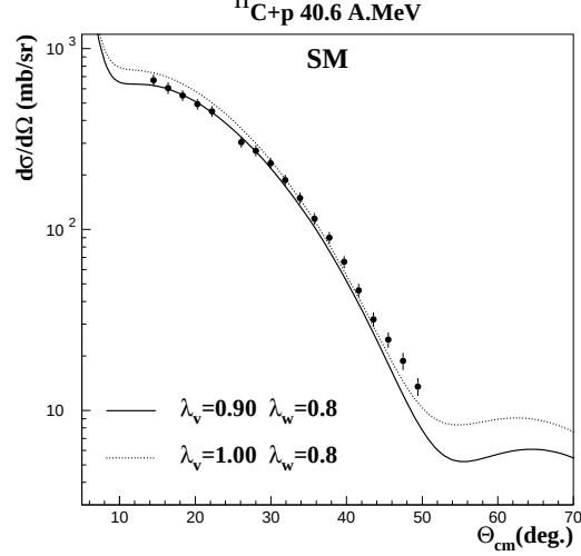
FIG. 4.19 – Distribution angulaire de la diffusion élastique ^{11}\text{C} + p à 40.6\text{ A.MeV} calculée avec le potentiel JLM (avec et sans normalisation de la partie réelle) et les densités SM. Les calculs sont comparés aux données.
