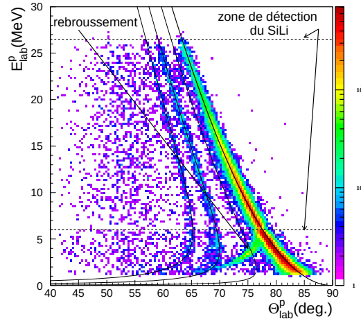
FIG. 3.13 – Matrice (\theta_{lab}^p; E_{lab}^p) pour la réaction ^{11}C + p à 40.6 A.MeV . La sélection des protons dans les deux premiers étages de MUST est prise en compte
