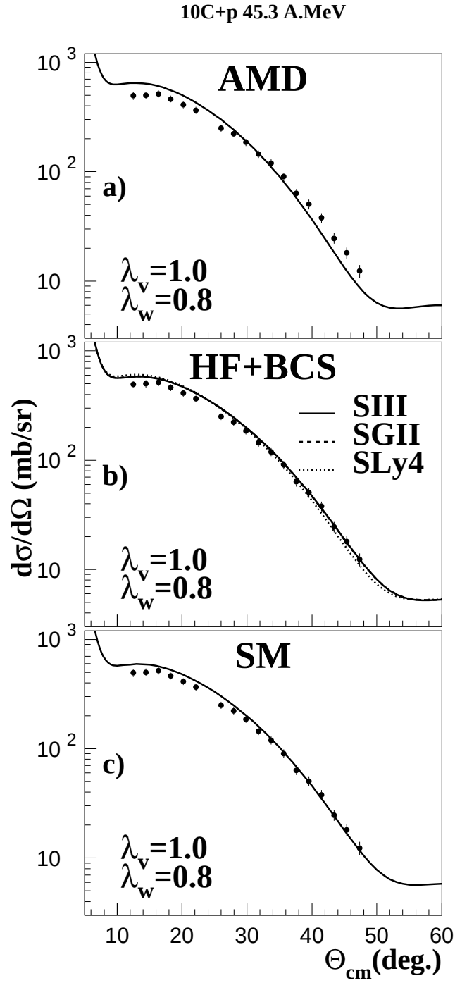
FIG. 4.7 – Distributions angulaires de la diffusion élastique ^{10}\text{C} + p à 45.3 A.MeV calculées avec le potentiel JLM (normalisation de la partie imaginaire \lambda_w = 0.8 ) et différentes densités. Les calculs sont comparés aux données.
