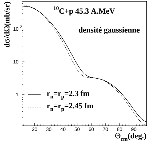
FIG. 1.9 – Influence du rayon carré moyen de la densité de matière sur la distribution angulaire avec le potentiel JLM
