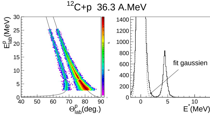
FIG. 3.23 – Matrice de corrélation (\theta_{lab}^p; E_{lab}^p) et spectre en énergie d'excitation pour la simulation de la réaction ^{12}C + p à 36.3 A.MeV avec une cible de 8.25 mg/cm^2
