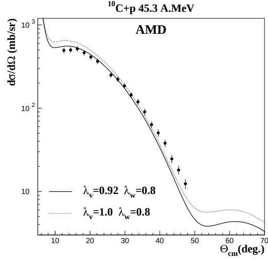
FIG. 4.8 – Distribution angulaire de la diffusion élastique ^{10}\text{C} + p à 45.3 \text{ A.MeV} calculée avec le potentiel JLM (avec et sans normalisation de la partie réelle) et les densités AMD. Les calculs sont comparés aux données.
