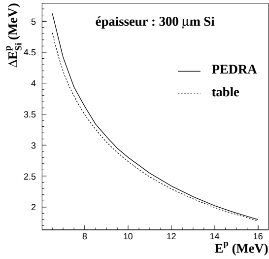
FIG. 3.4 – Pertes d’énergies pour des protons dans 300 \mu\text{m} de Silicium. Calculs effectués à partir d’une table de pertes d’énergie et d’un calcul analytique (programme PEDRA ).
