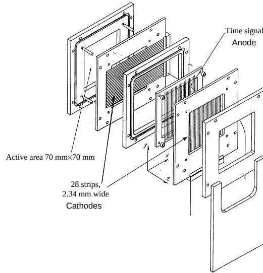
FIG. 2.8 – composition du détecteur CATS
