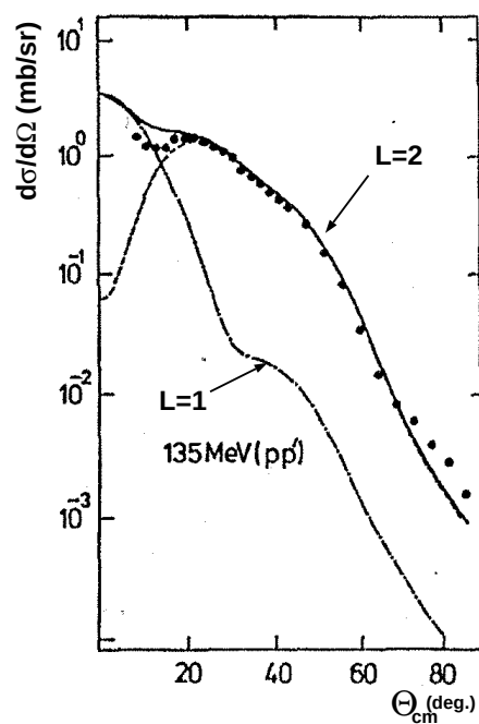
FIG. 4.29 – Diffusion inélastique vers le premier état 3/2^- à 3.68\text{ MeV} du ^{13}\text{C} en cinématique directe avec un faisceau de protons de 135\text{ MeV} . Comparaison avec des calculs effectués pour différentes nature de transition ( L = 1 et L = 2 ) [116]
