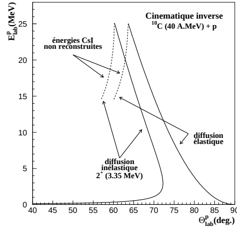
FIG. 3.7 – Cinématique du proton de recul pour la réaction en cinématique inverse ^{10}\text{C} sur proton à 40\text{ A.MeV} . Diffusion élastique et diffusion inélastique vers le premier état excité à 3.35\text{ MeV} .
