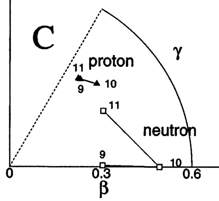
FIG. 1.6 – Déformations des distributions de neutrons et de protons pour les isotopes de carbone déficitaires en neutrons prédites par AMD [16]
