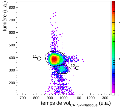
FIG. 3.8 – Matrice d’identification des particules détectées dans une des lattes du Mur de plastique en coïncidence avec un proton dans un des modules de MUST .
