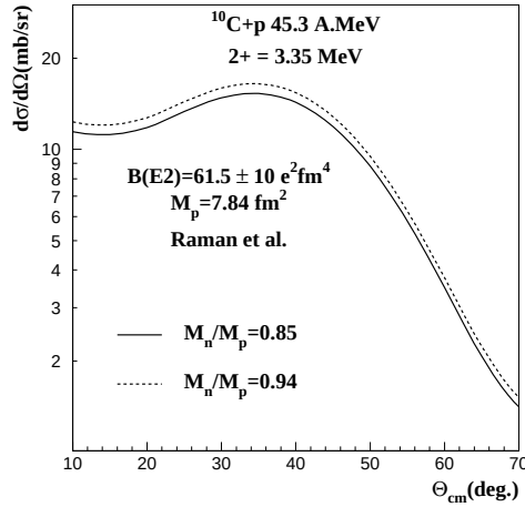
FIG. 1.11 – sensibilité de la distribution angulaire de section efficace de la diffusion inélastique ^{10}\text{C} + p à 45.3 \text{ A.MeV} vers le premier état 2^+ du ^{10}\text{C} à 3.35 \text{ MeV} au rapport M_n/M_p . M_p est fixé par la valeur expérimentale du B(E2) de la transition.
