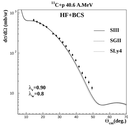
FIG. 4.21 – Distribution angulaire de la diffusion élastique ^{11}\text{C} + p à 40.6 \text{ A.MeV} calculée avec le potentiel JLM (avec et sans normalisation de la partie réelle) et les densités HF+BCS. Les calculs sont comparés aux données.
