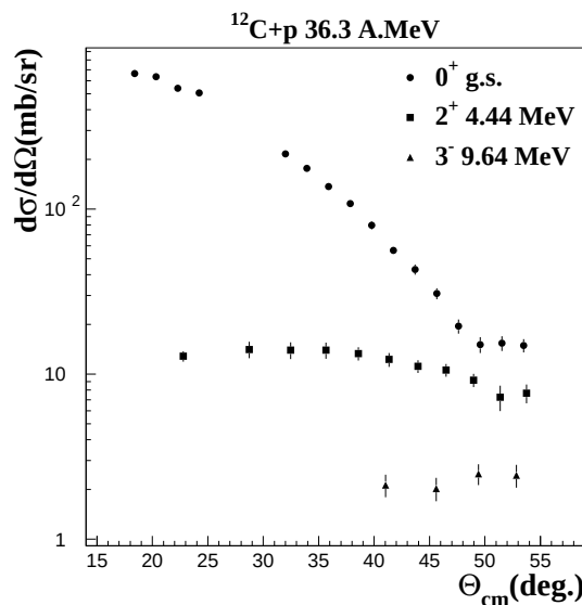
FIG. 3.26 – Distributions angulaires de section efficace pour les diffusions élastique et inélastique vers les 2^+ et 3^- à 4.44 MeV et 9.64 MeV
