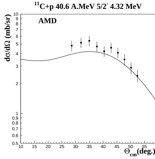
FIG. 4.24 – Diffusion inélastique vers le premier état 5/2^- à 4.32 \text{ MeV} du ^{11}\text{C} . La courbe correspond au calcul effectué avec les densités AMD.
