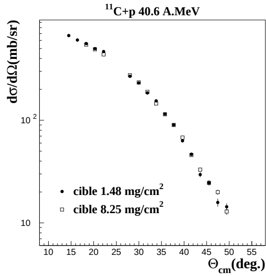
FIG. 3.28 – Comparaison des distributions angulaires de section efficace de la diffusion ^{11}\text{C}+ à 40.6 \text{ A.MeV} pour les deux cibles de polypropylène ( 1.48 \text{ mg/cm}^2 et 8.25 \text{ mg/cm}^2 )
