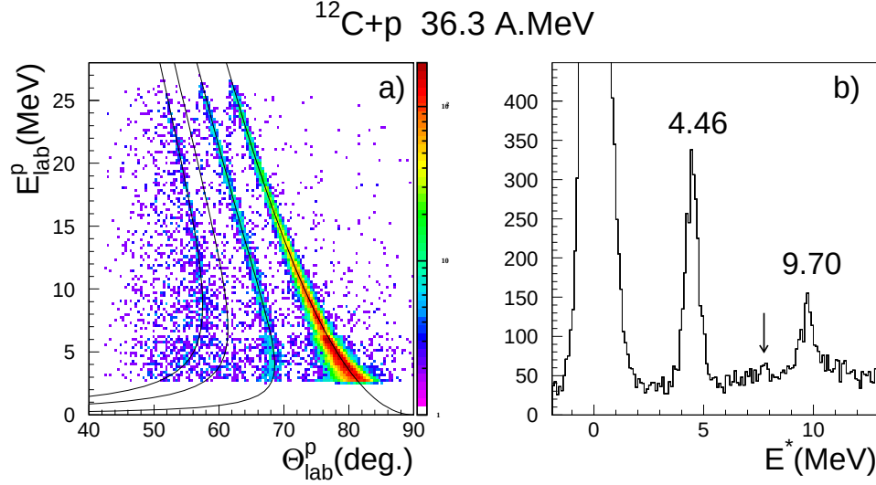
FIG. 3.15 – Matrice de corrélation (\theta_{\text{lab}}^p; E_{\text{lab}}^p) et spectre en énergie d'excitation du ^{12}\text{C} pour la réaction ^{12}\text{C} + p à 36.3 A.MeV.
