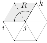
Fig. 4. The edge (i, j)_R precedes the edge (j, k)_R
