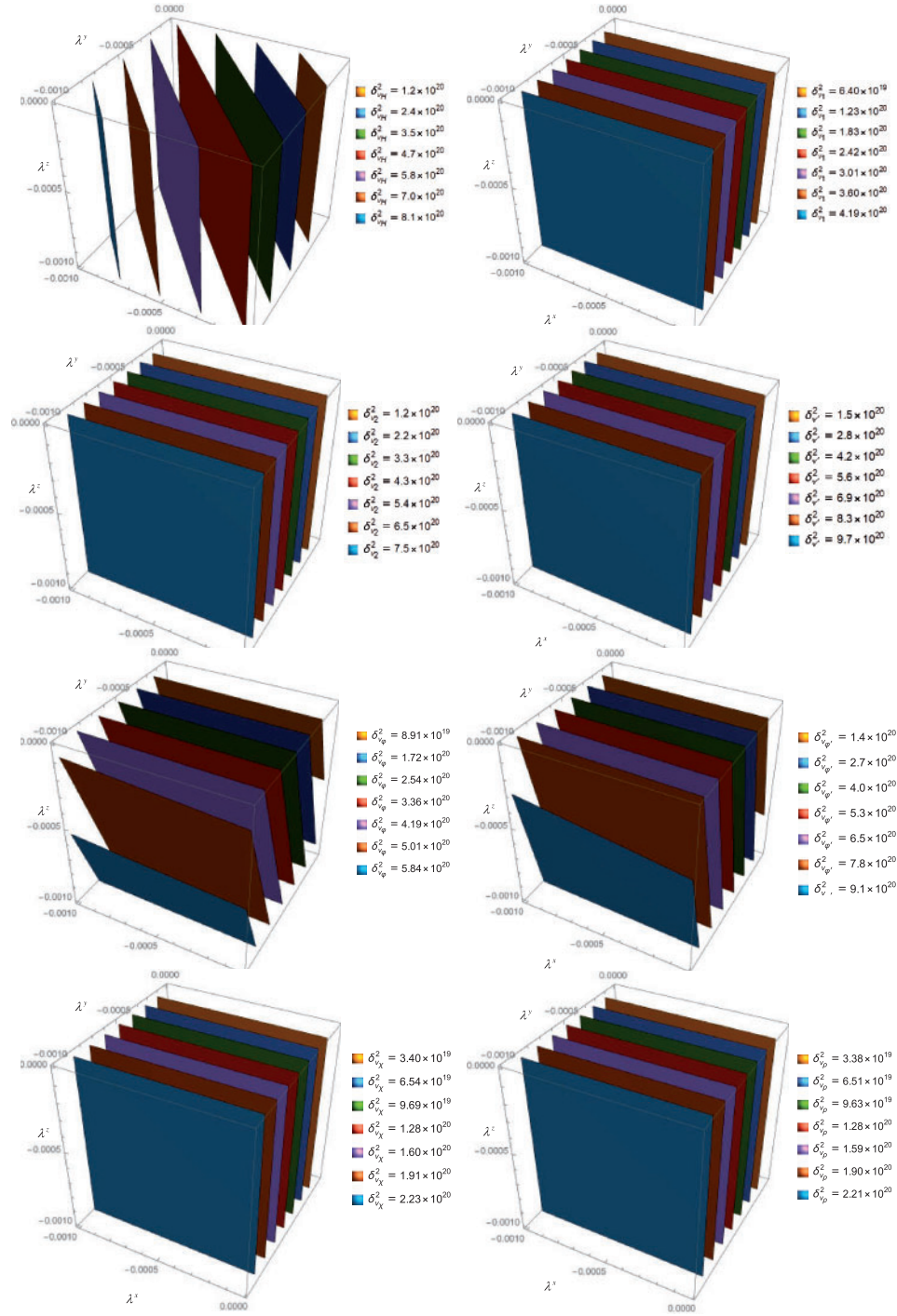
Fig. 1. \delta_{\nu_h}^2, \delta_{\nu_1}^2, \delta_{\nu_2}^2, \delta_{\nu_3}^2, \delta_{\nu_4}^2, \delta_{\nu_5}^2, \delta_{\nu_6}^2, \delta_{\nu_7}^2 vs. \lambda^x, \lambda^y , and \lambda^z with \lambda^x \in (-10^{-3}, -10^{-5}) , \lambda^y \in (-10^{-3}, -10^{-5}) , and \lambda^z \in (-10^{-3}, -10^{-5}) .
