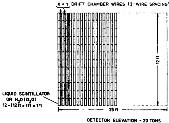
Fig. 7. Detector
