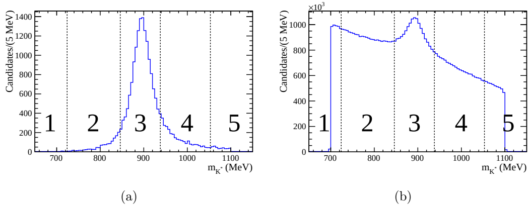
FIGURE 5 : Distribution de masse invariante du K^{*0} 2016 pour les évènements de signaux simulés (a) et données (b) pour l'état final 3\pi 3\pi . Les distributions pour l'autre état final et les autres années de prise de données sont similaires.
