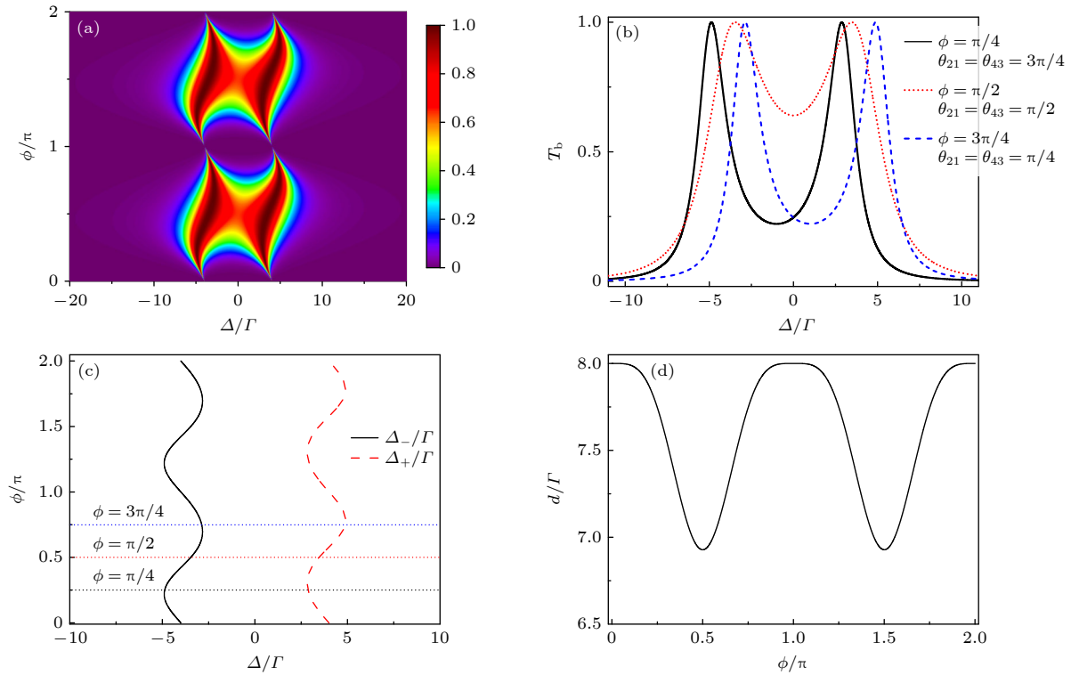
图 4 (a) 在局域耦合相位差 \theta_{21} = \theta_{43} = \pi - \phi 条件下 T_b 随失谐 \Delta 和累积相位 \phi 的变化; (b) 几个典型的累积相位 \phi 取值下与图 (a) 对应的单光子散射曲线图, 参数取值为: 黑色实线 \phi = \pi/4 , \theta_{21} = \theta_{43} = 3\pi/4 , 红色点线 \phi = \theta_{21} = \theta_{43} = \pi/2 , 蓝色虚线 \phi = 3\pi/4 , \theta_{21} = \theta_{43} = \pi/4 ; (c) 为图 (a) 中散射率最大值 T_b = 1 的轮廓图, 即单光子谱线中双峰的峰位 \Delta_{\pm} 随 \phi 的变化; (d) 双峰间距 d 随 \phi 的变化. 其他参数为: \lambda/\Gamma = 4
