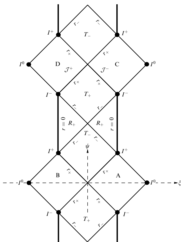
Рис. 7. Метрика Рейснера–Нордстрёма. А, В, С, D – асимптотически плоские вселенные, \psi — временная координата, \xi — пространственная координата, I^0 — пространственная бесконечность, I^+ — бесконечно будущее, I^- — бесконечно прошлое, T_+ — расширяющаяся T -область, T_- — сжимающаяся T -область, r = 0 — сингулярность пространства-времени, r_+ — горизонт событий, r_- — горизонт Коши.
