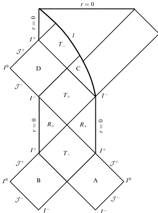
Рис. 11. Эволюция в С-вселенной оболочки I , содержащей внутри себя метрику Крускала (в верхней правой части рисунка). Эта эволюция не является следствием событий во вселенной A . Обозначения те же, что и на предыдущих рисунках.
