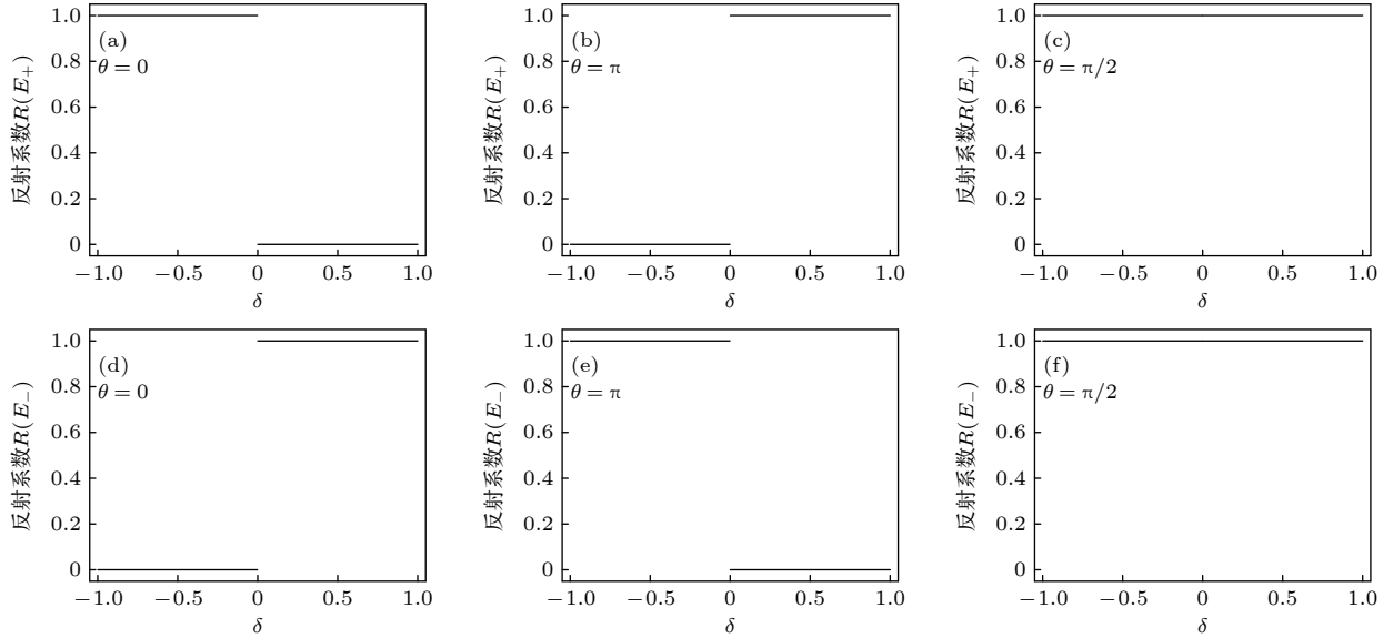
图4 反射系数 R 随 \delta 的变化 (a)–(c) 单光子能量为 E_+ 时, 反射系数 R 随 \delta 的变化; (d)–(f) 单光子能量为 E_- 时, 反射系数 R 随 \delta 的变化; 其他参数设置为 \Delta = 0 , k = \pi , J_a = J_b = J = 1 . 人工规范场相位 \theta 具体取值为 (a), (d) \theta = 0 ; (b), (e) \theta = \pi ; (c), (f) \theta = \pi/2
