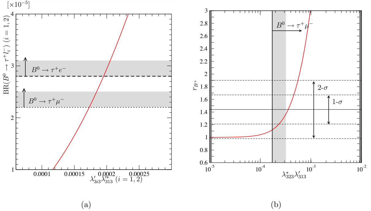
図 3.15: (a) は RPV 結合定数の関数としての B^0 \rightarrow \tau^+ l_i^- ( i = 1, 2 ) 過程の分岐比を描いた。横のラインはそれぞれ破線が \text{BR}(B^0 \rightarrow \tau^+ e^-) の実験データによる許容上限値、点線が \text{BR}(B^0 \rightarrow \tau^+ \mu^-) の実験データによる許容上限値である。(b) は荷電スカラータウレプトンの s -チャンネル交換ダイアグラムにおける、パラメータ r_{B^+} へのレプトンフレーバーを破る寄与を描いた。横軸が RPV 結合定数、縦軸がパラメータ r_{B^+} で、縦線は B^0 \rightarrow \tau^+ \mu^- 過程における実験値から求めた許容上限値を表している。横の実線と破線はそれぞれ (3.27) 式、 r_{B^+} の中心値と 1\sigma の値、 2\sigma の値を表す。
