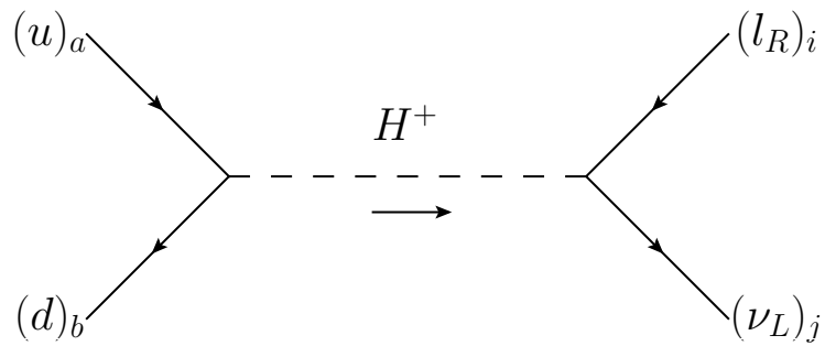
図 3.3: 荷電ヒッグスボソンを介した P \rightarrow l_i^+ \nu_j ( P = D_s^+ or B^+ ) 過程のダイアグラムを描いた。 a, b, i, j は各粒子の世代を表す。 D_s^+ \rightarrow \tau^+ \nu 過程のとき a = 2, b = 2, i = 3, j = 3 で, B^+ \rightarrow \tau^+ \nu 過程のとき a = 1, b = 3, i = 3, j = 3 である。
