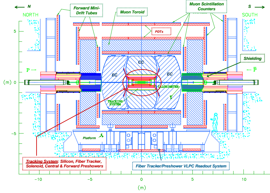
Fig. 8. D0 detector
