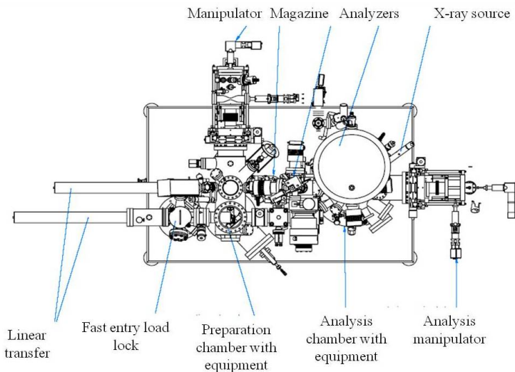
Fig. 6. UHV target chamber.
