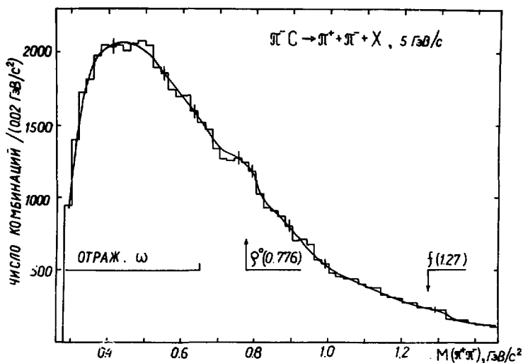
Рис.1. Инклюзивный спектр эффективных масс пар ( \pi^+\pi^- )-мезонов в \pi^-C -взаимодействиях при 5 ГэВ/с. Сплошная кривая - результат аппроксимации.
