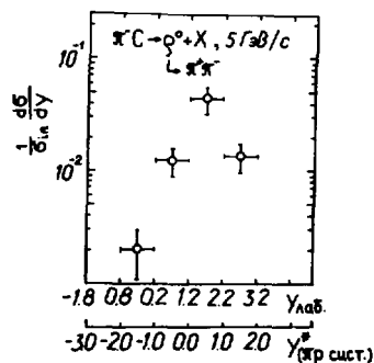
Рис.3. Распределение \rho^0 -мезонов по быстроте.
