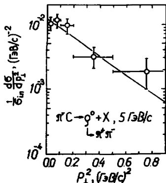
Рис.2. Распределение \rho^0 -мезонов по P_1^2 .
