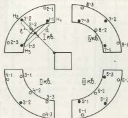
Рис. 4. Схематическое изображение квадрантов синхрофазотрона и расположение гидростатических датчиков.
