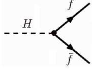
FIG. 1.6: Diagramme de Feynman du Higgs en fermions.
