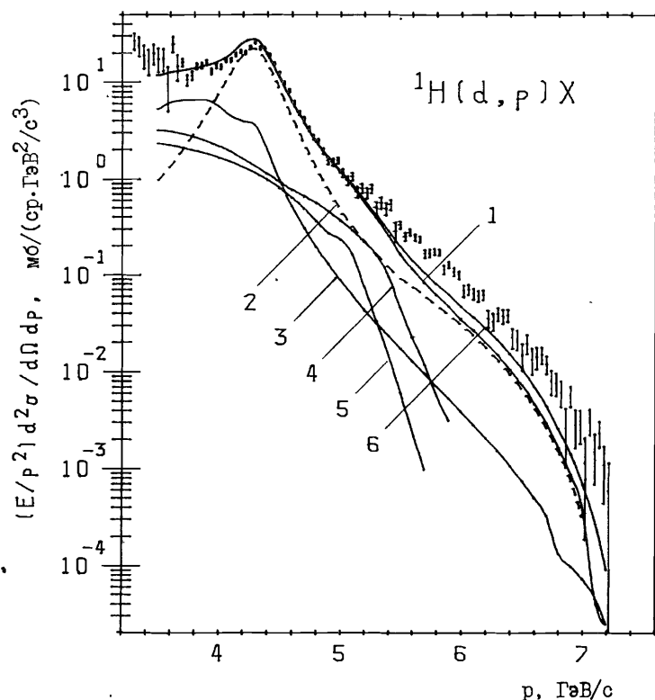
Рис. 4. То же, что и на рис. 3. Штриховая кривая 2 – вклад диаграммы рис. 1 с упругим рассеянием в нижней вершине, вычисленный со структурной функцией для парижского потенциала, кривая 3 – вклад неупругих процессов в нижней вершине диаграммы рис. 1, кривые 4 и 5 – вклады диаграмм рис. 2а и рис. 2б, кривая 1 – сумма всех указанных вкладов, кривая 6 – сумма этих же вкладов в случае вычислений со структурной функцией для потенциала Рейда.
