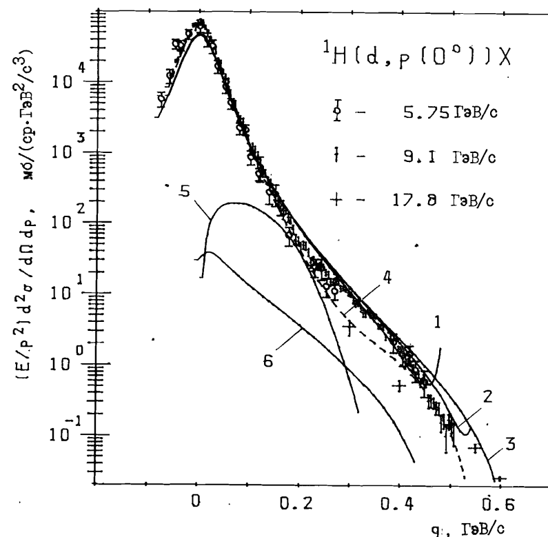
Рис. 5. Импульсные спектры протонов, испущенных под 0^\circ в реакции {}^1\text{H}(d, p)X при 5,75 /12/ , 9,1 /13/ и 17,8 ГэВ/с /20/ , в системе покоя дейтрона. Кривые 1, 2 и 3 – результаты расчетов по формуле (6) для начальных импульсов дейтронов 5,75, 9,1 и 17,8 ГэВ/с, соответственно, со структурной функцией работы /17/ . Кривая 4 – расчет при 9,1 ГэВ/с с "нерелятивистской" структурной функцией, полученной из волновой функции дейтрона для парижского потенциала. Кривые 5 и 6 – вклады диаграмм рис. 2а и рис. 2б при 9,1 ГэВ/с.
