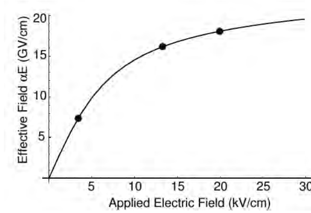
Figure F.2 – Facteur d’amplification pour YbF [SAHH06].
