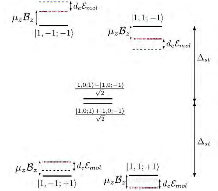
Figure F.3 – Structure de niveaux d'énergie de ThO dans l'état ^3\Delta_1(J = 1) dans des champs électrique et magnétique appliqués [VCG + ].
