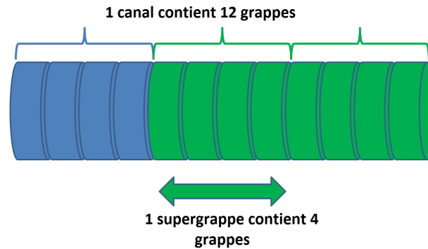
FIGURE III.1.2 – Constitution d'un canal de réacteur CANDU
