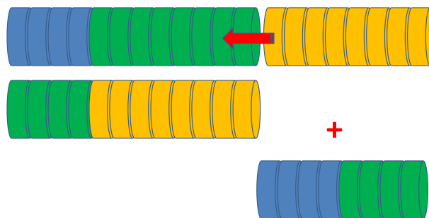
FIGURE III.1.4 – Principe de renouvellement de combustible par canal : à l'équilibre, 4 grappes proviennent du chargement N-2 (bleu) et 8 du chargement N-1 (vert). Le rechargement N (orange) consiste à "pousser" 8 grappes à l'autre bout du canal. On récupère alors les 4 grappes du rechargement N-2 et 4 grappes du rechargement N-1. Restent en réacteur 4 grappes du rechargement N-1 et les 8 nouvelles grappes.
