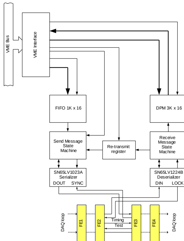
Fig. 7 DAQ loop test module
