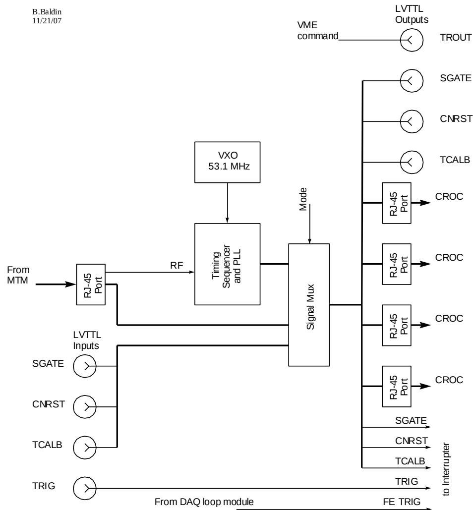
Fig. 6 Timing module
