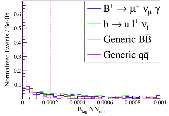
(d) Muon channel in the sub-range.
