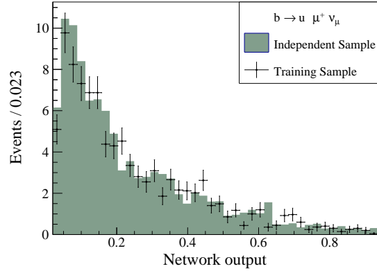
(d) Muon channel b \rightarrow u \ell^+ \nu_\ell MC.
