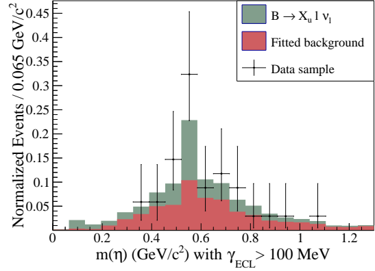
(d) Muon channel: B \rightarrow X_u \ell^+ \nu_\ell enriched SB.
