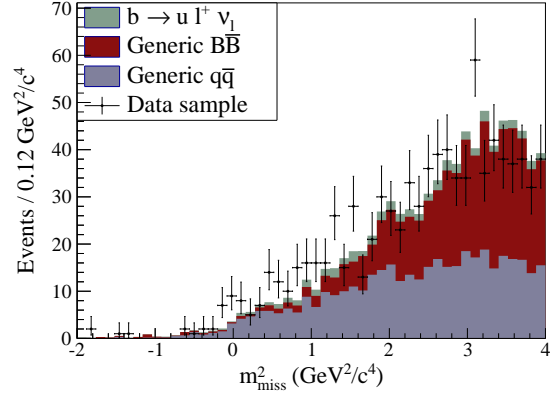
(d) Electron channel.
