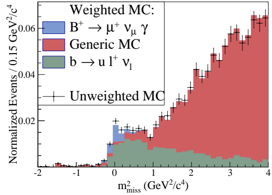
(d) Muon channel normalized.
