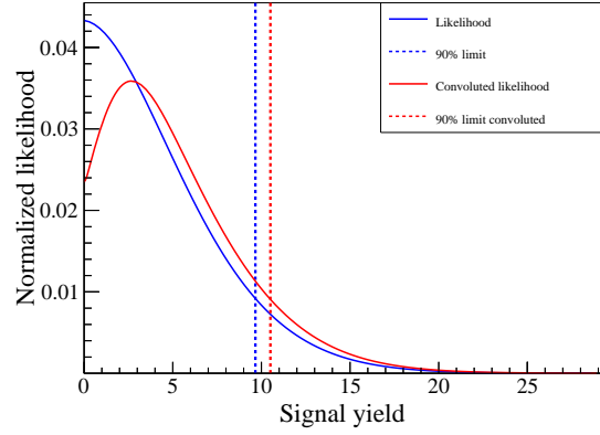
(d) Muon channel of the secondary analysis.
