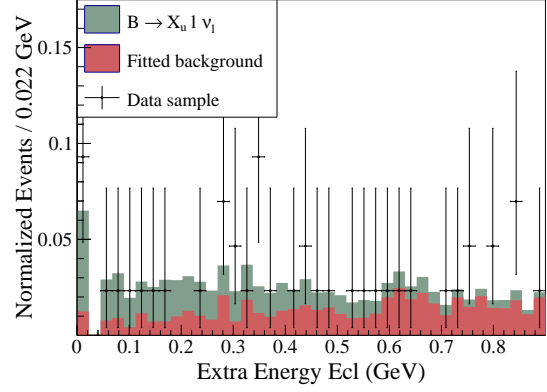
(d) Muon channel: B \rightarrow X_u \ell^+ \nu_\ell enriched SB.
