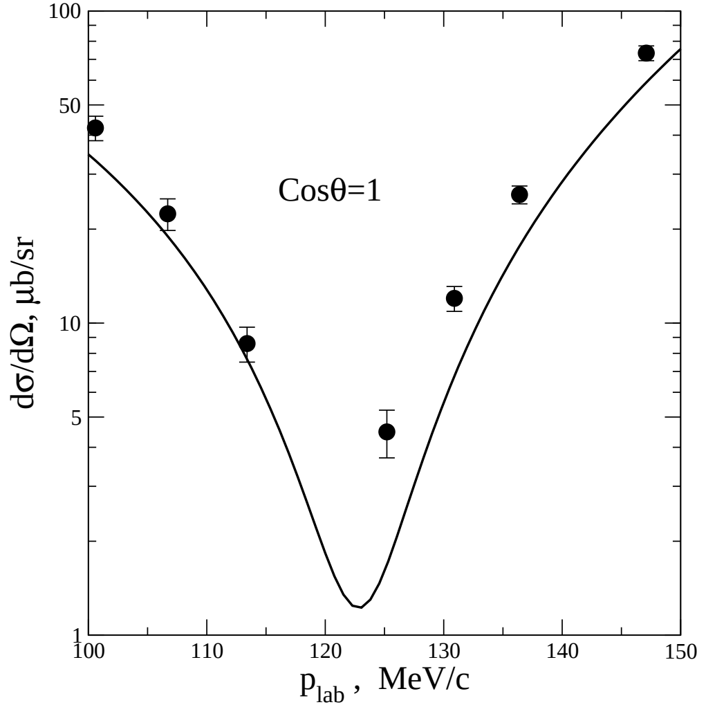
Рис. 1.6. Деструктивная интерференция s - и p -волн. Дифференциальное сечение d\sigma/d\Omega реакции одиночной перезарядки \pi^- p \rightarrow \pi^0 n как функция импульса налетающего пиона p_{lab} при угле вылета \theta = 0 . На рисунке представлены результаты расчета с параметризацией фазовых сдвигов (1.15) (сплошная линия) в сравнении с экспериментальными данными [22].
