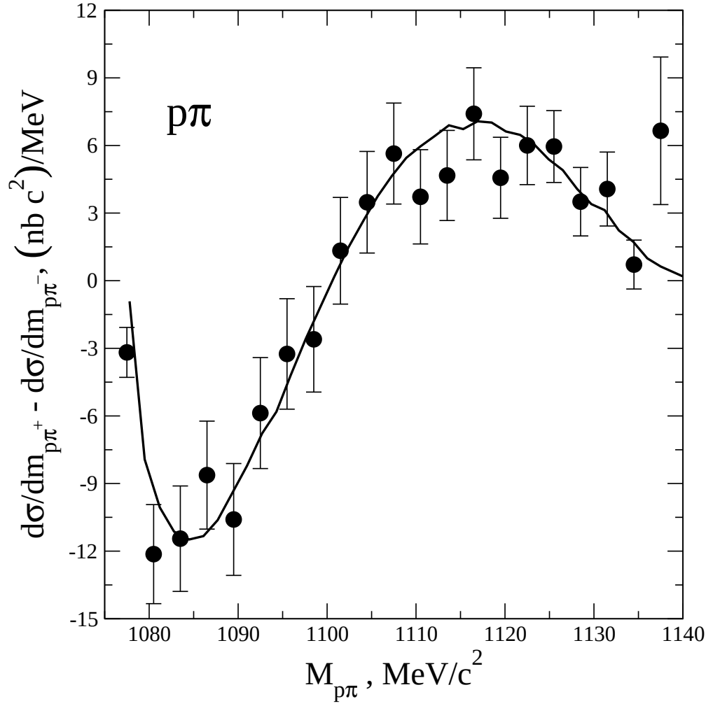
Рис. 3.5. Асимметрия (d\sigma/dm_{p\pi})_{\pm} ( \text{nb} \cdot c^2/\text{MeV} ) реакции pp \rightarrow pp\pi^+\pi^- как функция инвариантной массы M_{p\pi} системы протон - пион. Сплошная линия – результаты численных расчетов с амплитудой (3.12), жирные точки – экспериментальные данные CELSIUS [14].
