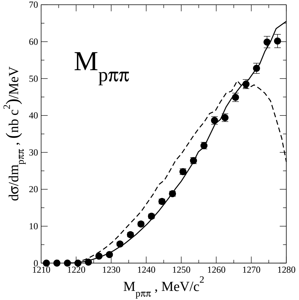
Рис. 3.11. Спектр инвариантной массы системы r\pi\pi для реакции pr \rightarrow pr\pi^+\pi^- . Сплошной линией изображены результаты расчета с амплитудой (3.12), учитывающей NN взаимодействие в конечном состоянии в приближении эффективного радиуса. Жирные точки – экспериментальные данные CELSIUS [14]. Для сравнения пунктирной линией изображен фазовый объем.
