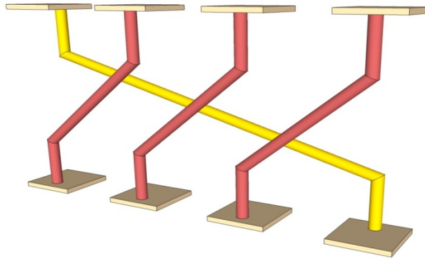
Figure 26. Diagonal vias.
