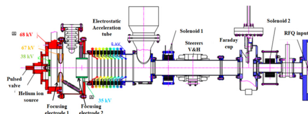
Fig. 6: LEBT layout.
